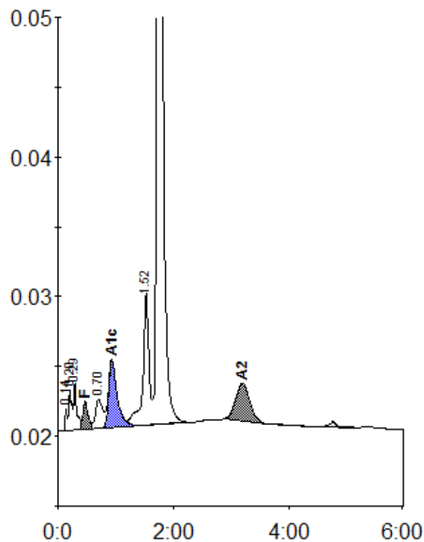
Peak table - ID: A0272607
