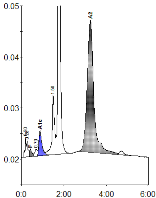
Peak table - ID: A1703398
