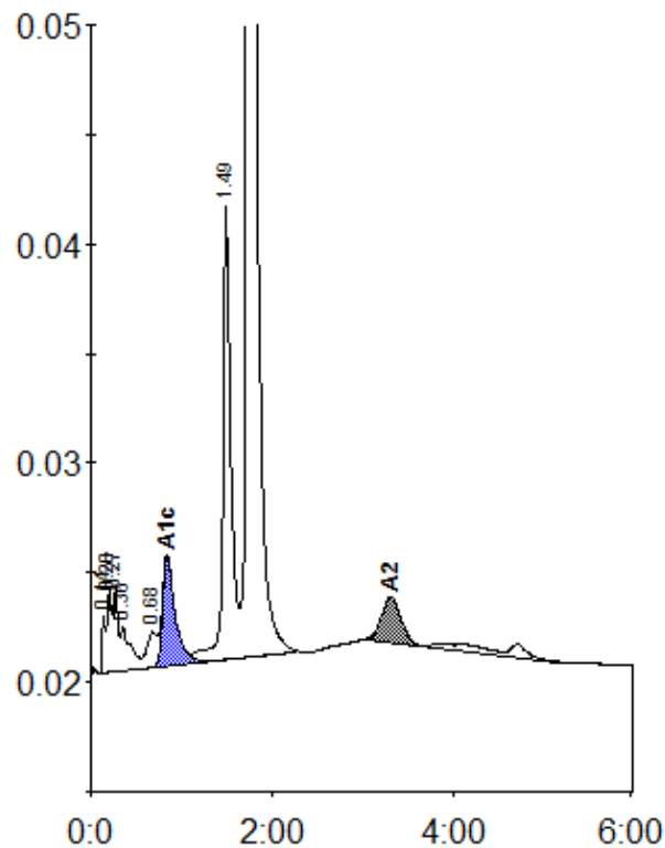
Peak table - ID: A2201164
