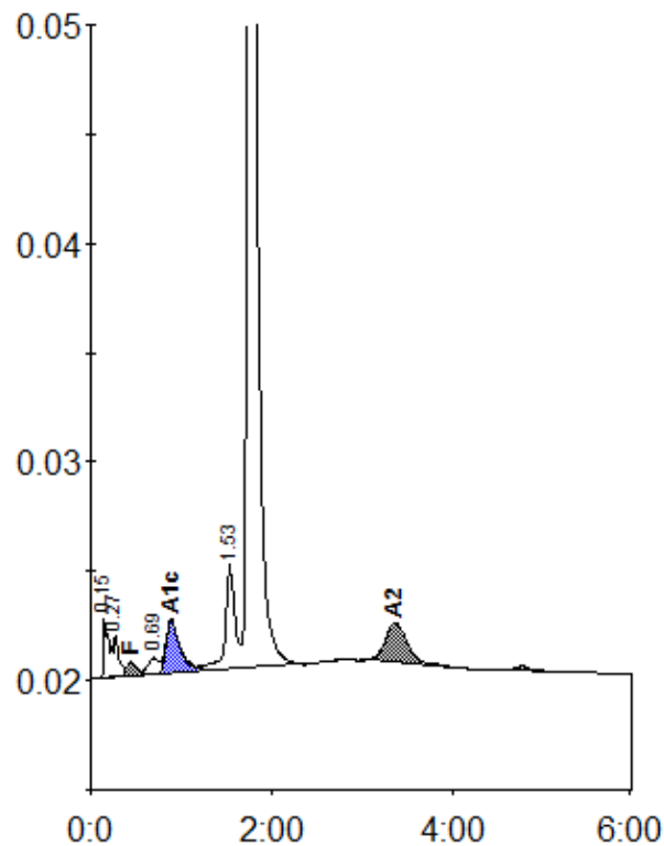
Peak table - ID: B2497759
