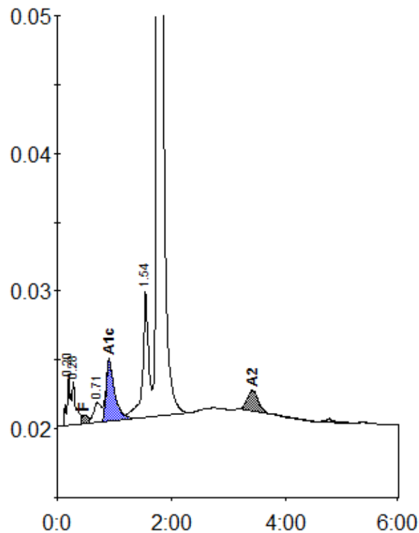
Peak table - ID: A2196083
