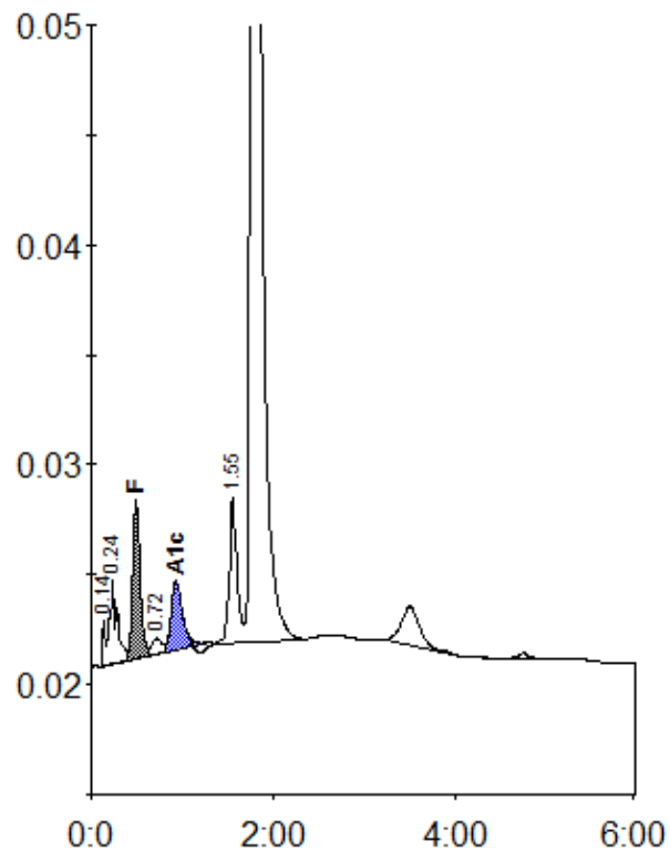
Peak table - ID: B2917550
